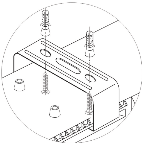
Рисунок 1. Монтаж изделия
